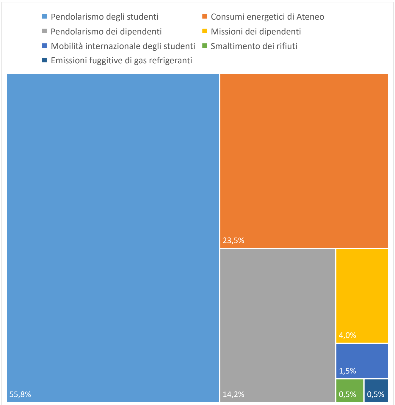
Figura 1 Ripartizione percentuale delle emissioni di gas serra dell'Università di Padova - anno 2019.
